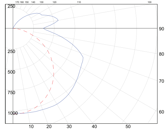
0° ——— Candela Plot 4Lamp T8 90° ———
