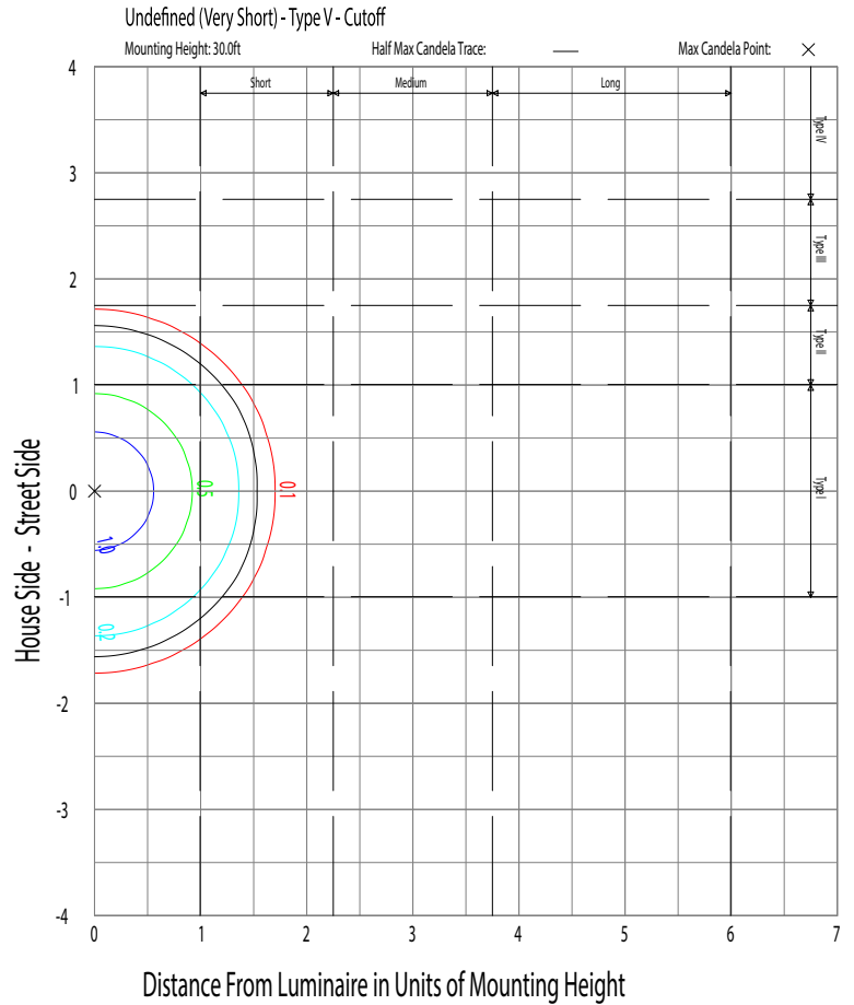
Iso-illuminance Plot
